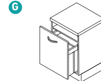
Unterschrank mit Wäschesortierung Höhe = 711 mm Breite = 600 mm 1 Auszug 2 Wäschekörbe 33 Liter 1 Behälter mit Deckel 20 Liter 1 Behälter 2,5 Liter Base cabinet with laundry sorting system Height = 711 mm Width = 600 mm 1 pull-out 2x 33 litre laundry baskets 1x 20 litre container with lid 1x 2.5 litre container
