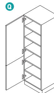
Seitenschrank Höhe = 1587, 1907, 2051, 2195 mm Breite = 600 mm 1 Drehtür verstellbare Fachböden 1 fester Fachboden Side cabinet Height = 1587, 1907, 2051, 2195 mm Width = 600 mm 1 hinge door Adjustable shelves 1 fixed shelf
