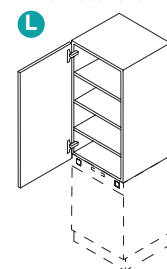
Aufsatzschrank Höhe = 1181 mm 1 Drehtür 3 verstellbare Fachböden Top-mounted cabinet Height = 1181 mm 1 hinge door 3 adjustable shelves
