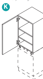
Aufsatzschrank Höhe = 861 mm 1 Drehtür 2 verstellbare Fachböden Top-mounted cabinet Height = 861 mm 1 hinge door 2 adjustable shelves
