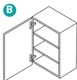
Hängeschrank Höhe = 579, 723, 867 mm Breite = 600 mm 1 Drehtür verstellbarer Fachboden Wall cabinet Height = 579, 723, 867 mm Width = 600 mm 1 hinge door adjustable shelf
